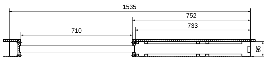
VAAKALEIKKAUS 1:15 SEINÄRUNKO; LIUKUOVIELEMENTTI, LEVYTYKSET, OVILEVY JA KARMIT
