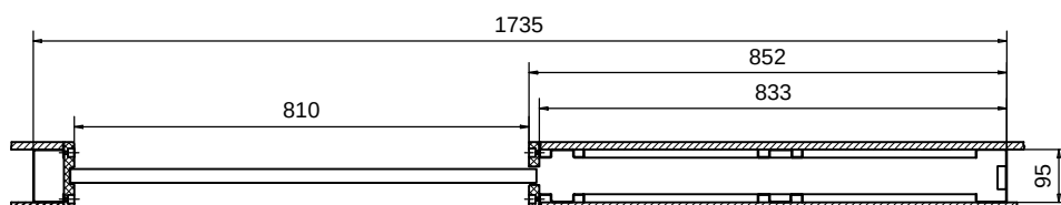
VAAKALEIKKAUS 1:15 SEINÄRUNKO; LIUKUOVIELEMENTTI, LEVYTYKSET, OVILEVY JA KARMIT
