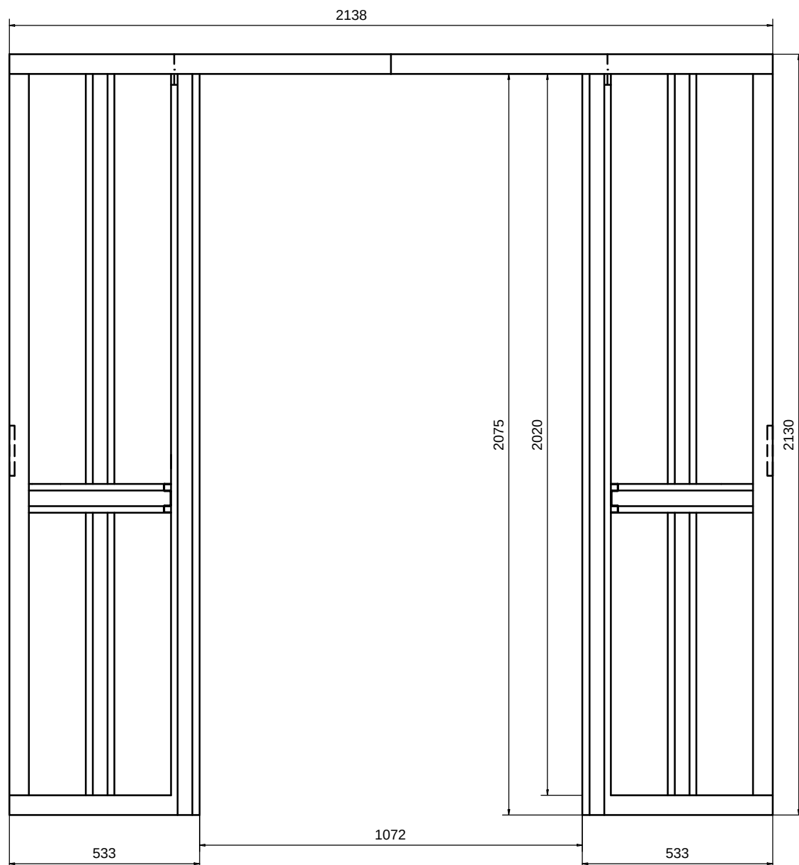
NAAMAKUVA 1:15 LIUKUOVIELEMENTTI LiO10PO
