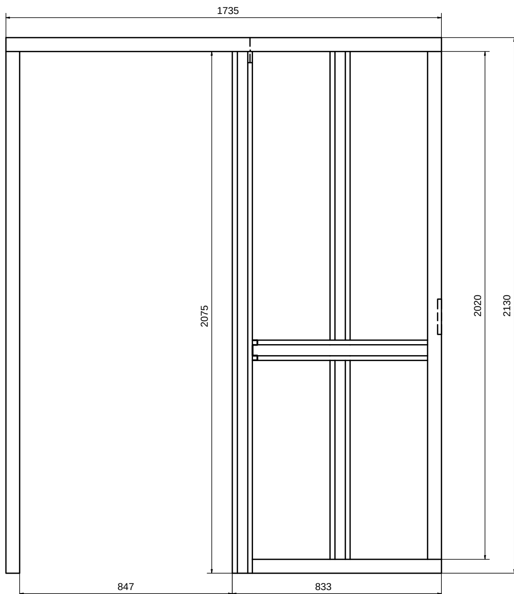
NAAMAKUVA 1:15 LIUKUOVIELEMENTTI LiO8
