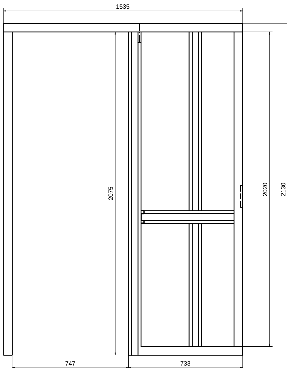
NAAMAKUVA 1:15 LIUKUOVIELEMENTTI LiO7
