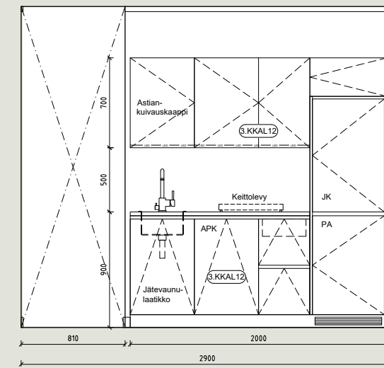
P4 Keittiötila/ Oleskelu 1:25 Army
