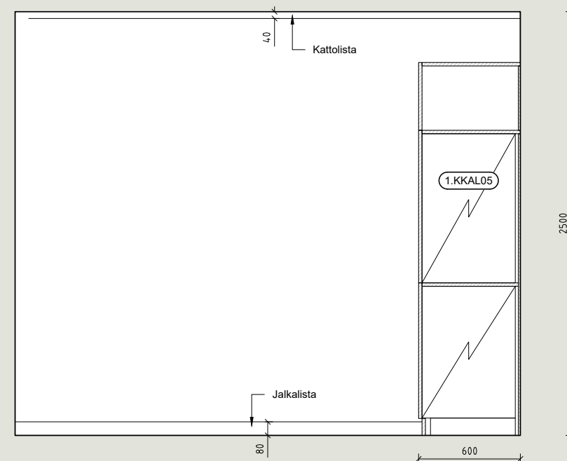
P16 S-MODUULI 1:25 Keittiö
