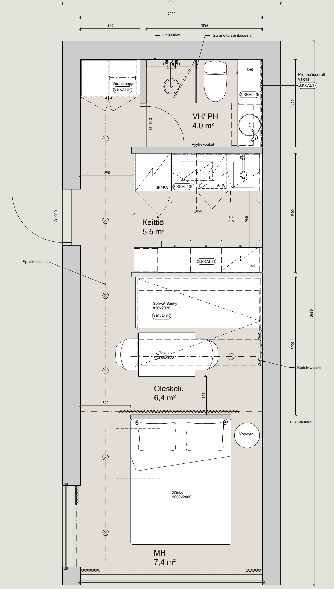
L- MODUULI HELMI KERROSALA 30,2 m 2
