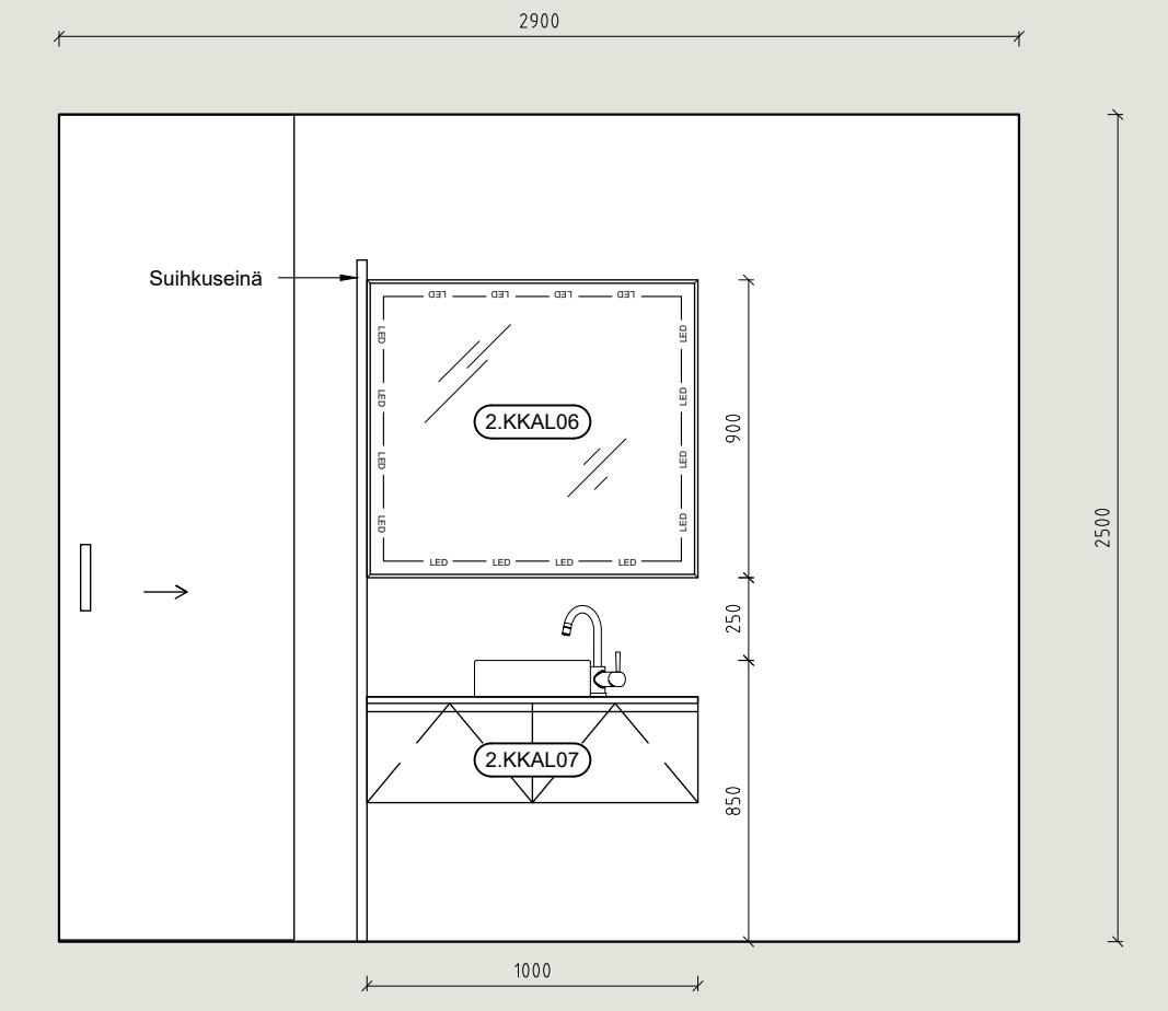
P16 M-MODUULI 1:25 Makuuhuone + WC
