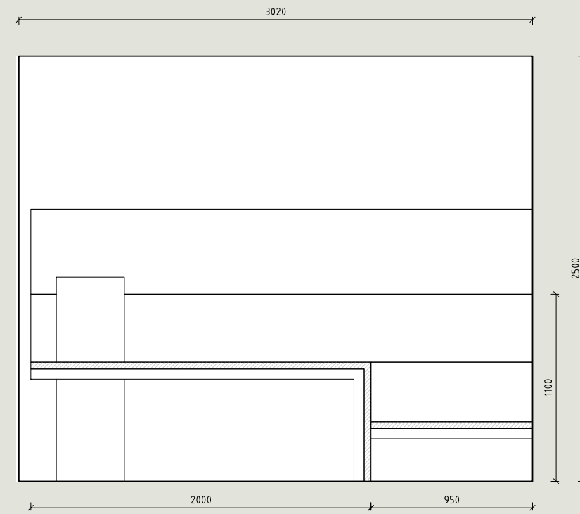
P12 S-MODUULI 1:25 Sauna
