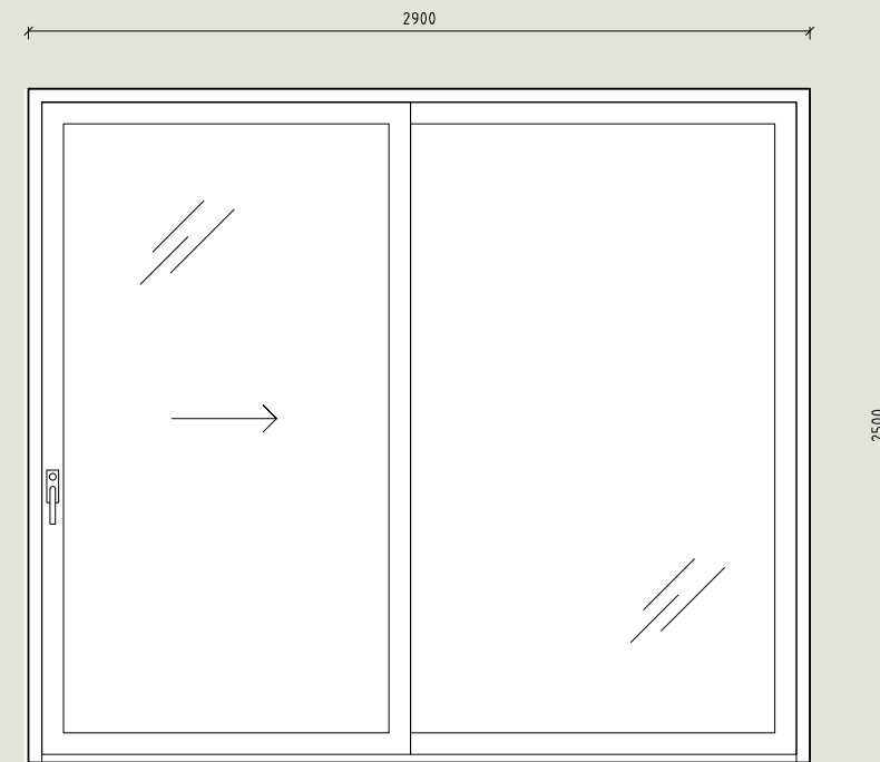
P1 S-MODUULI 1:25 Oleskelutila
