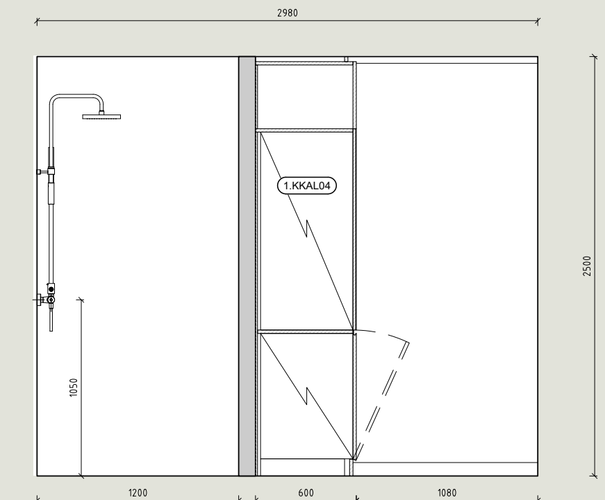
P8 S-MODUULI 1:25 Keittiö ja WC
