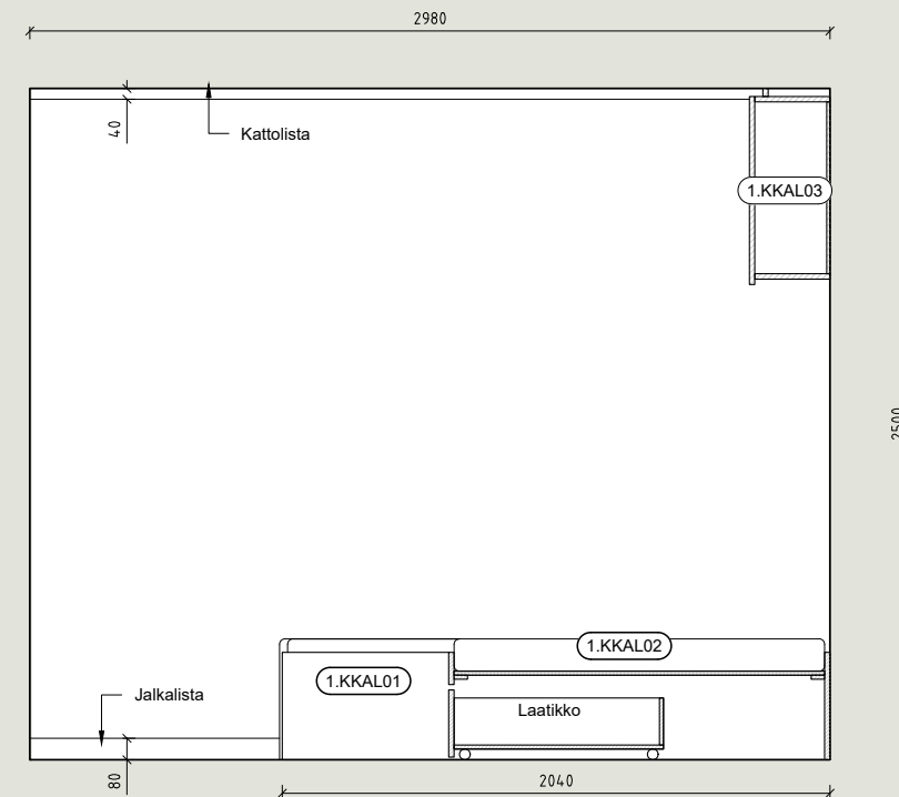
P2 S-MODUULI 1:25 Oleskelutila
