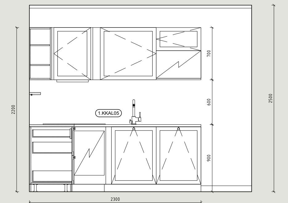
P18 S-MODUULI 1:25 Keittiö
