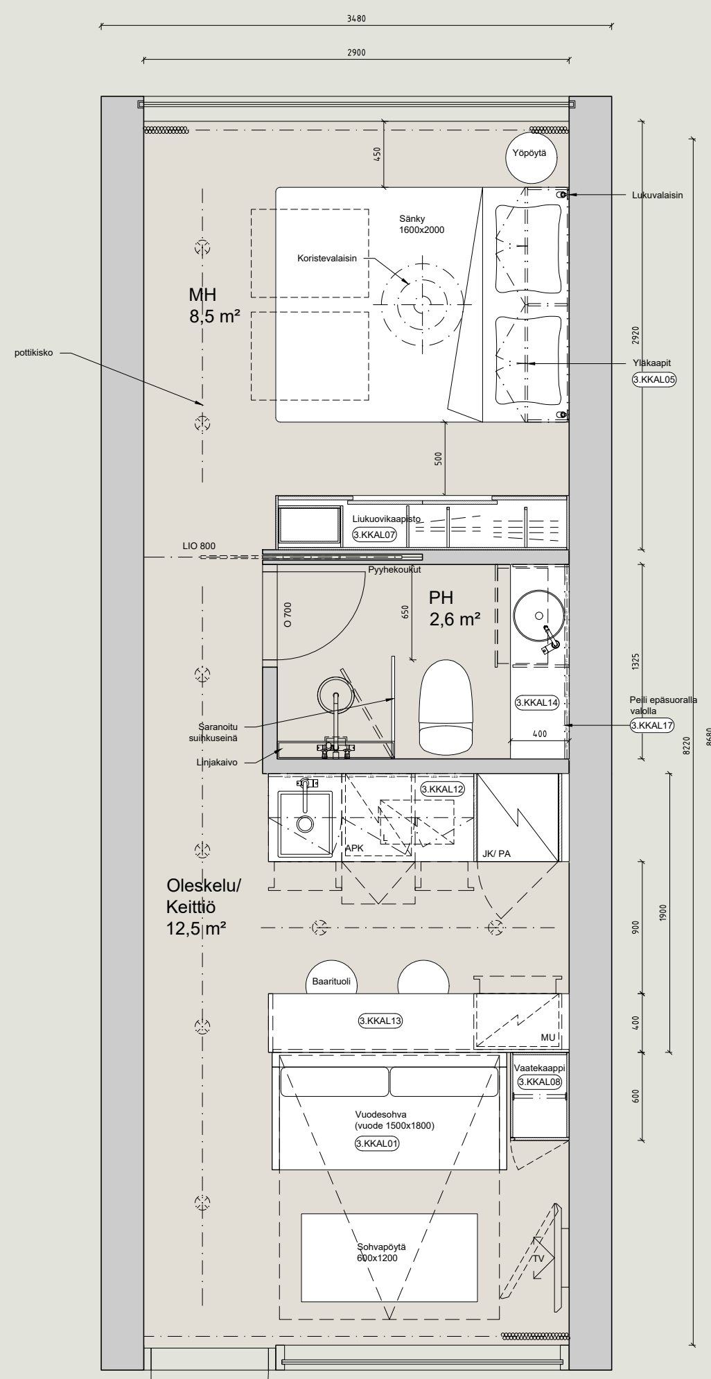
L- MODUULI ARMY KERROSALA 30,2 m 2
