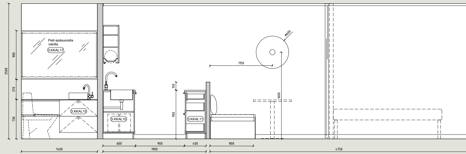
P2 Pesuhuone, keittiö, Oleskelu/Ruokailu Helmi
