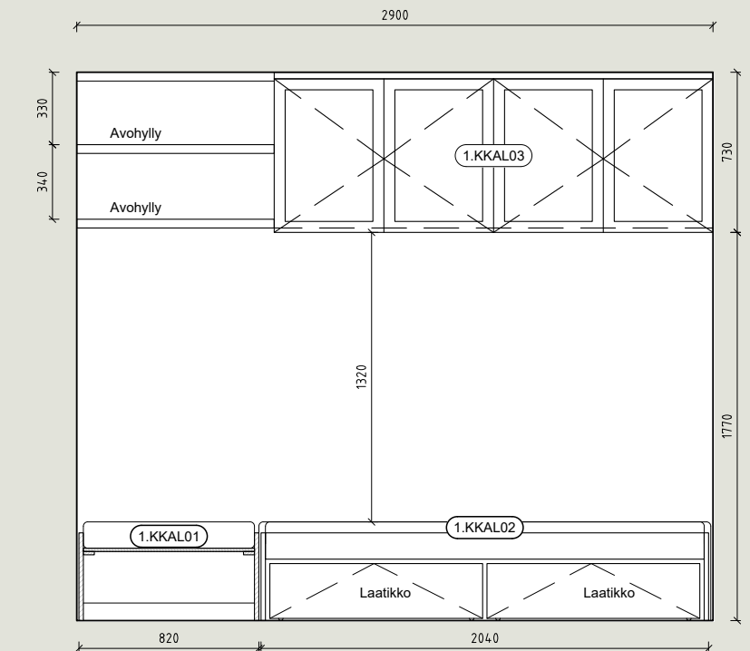
P3 S-MODUULI 1:25 Oleskelutila
