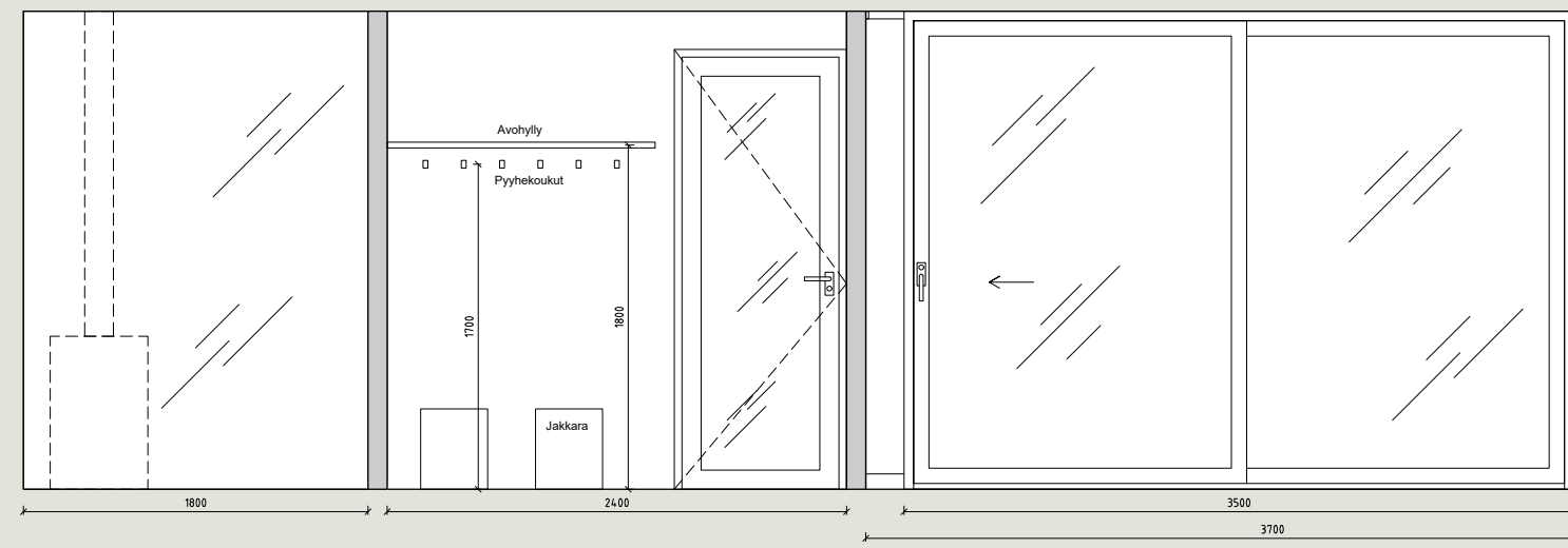
P1 Sauna, pesuhuone, oleskelutila Sauna 1:25
