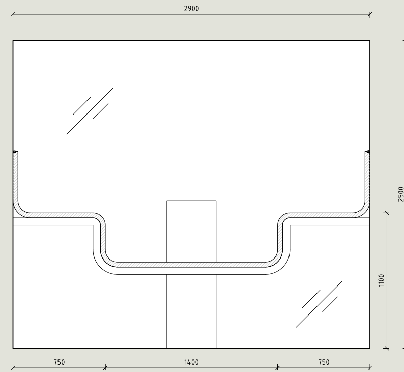
P11 S-MODUULI 1:25 Sauna isolla ikkunalla
