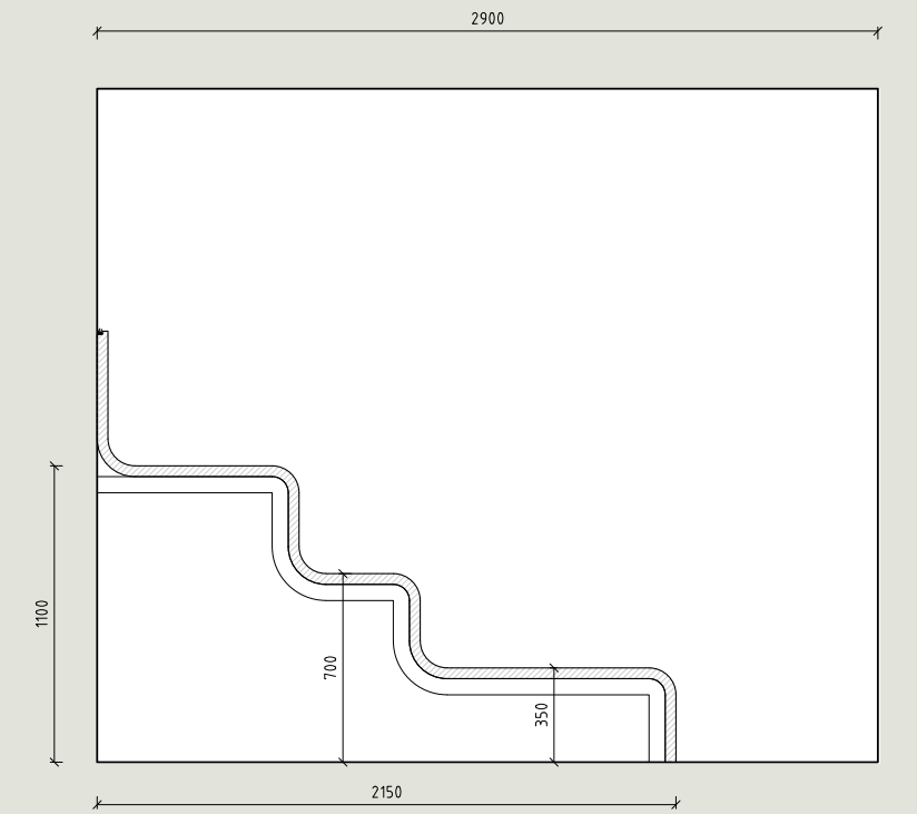
P13 S-MODUULI 1:25 Sauna
