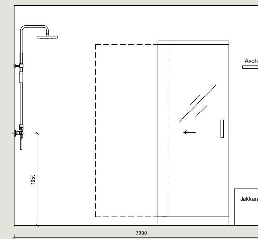
P6 Pesuhuone Sauna 1:25
