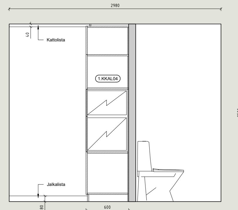
P6 S-MODUULI 1:25 Keittiö ja WC
