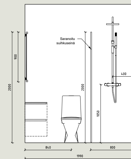
P9 Pesuhuone 1:25 Army
