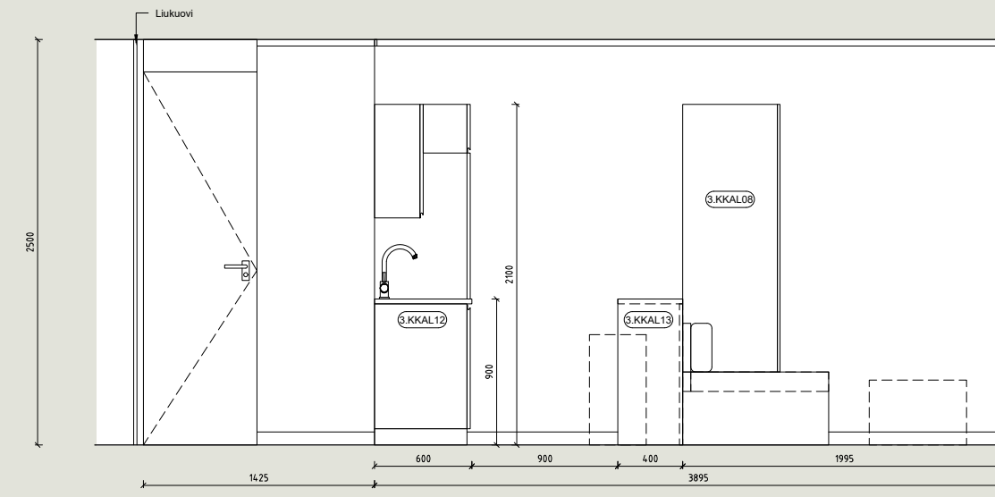
P3 Käytävä 1:25 Army
