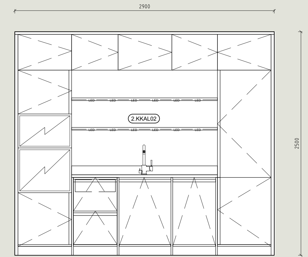
P9 M-MODUULI 1:25 Keittiö + ruokailutila
