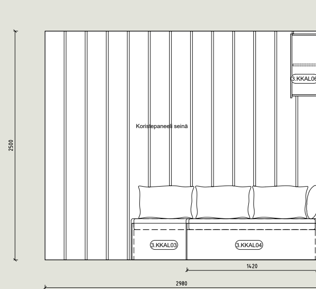
P3 Oleskelutila Sauna 1:25
