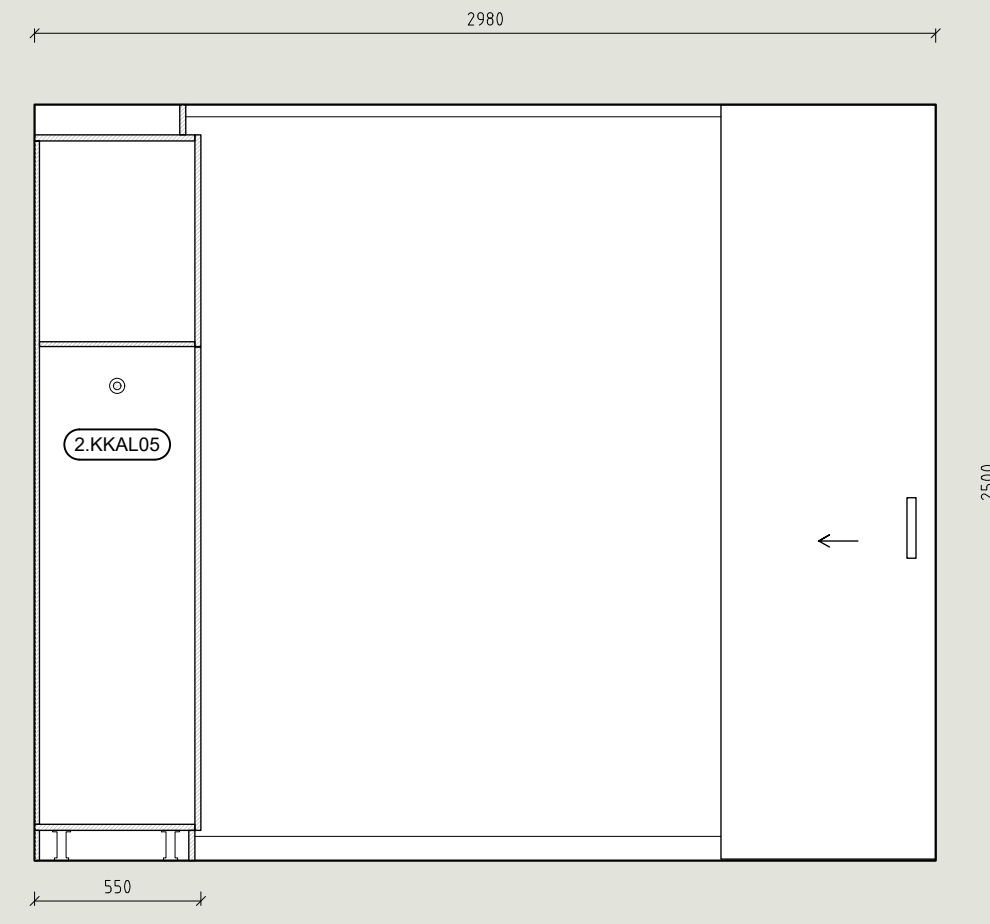
P15 M-MODUULI 1:25 Makuuhuone + WC
