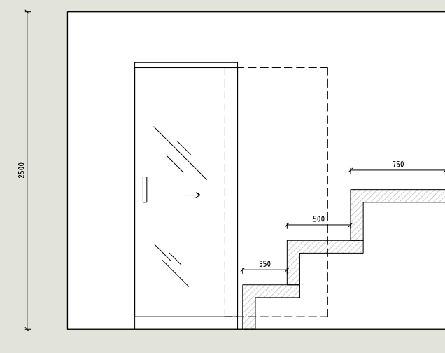
P11 Sauna Sauna 1:25
