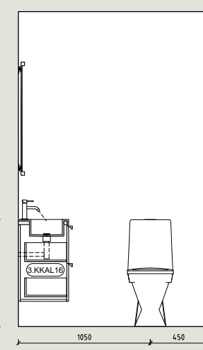
P9 WC Sauna 1:25
