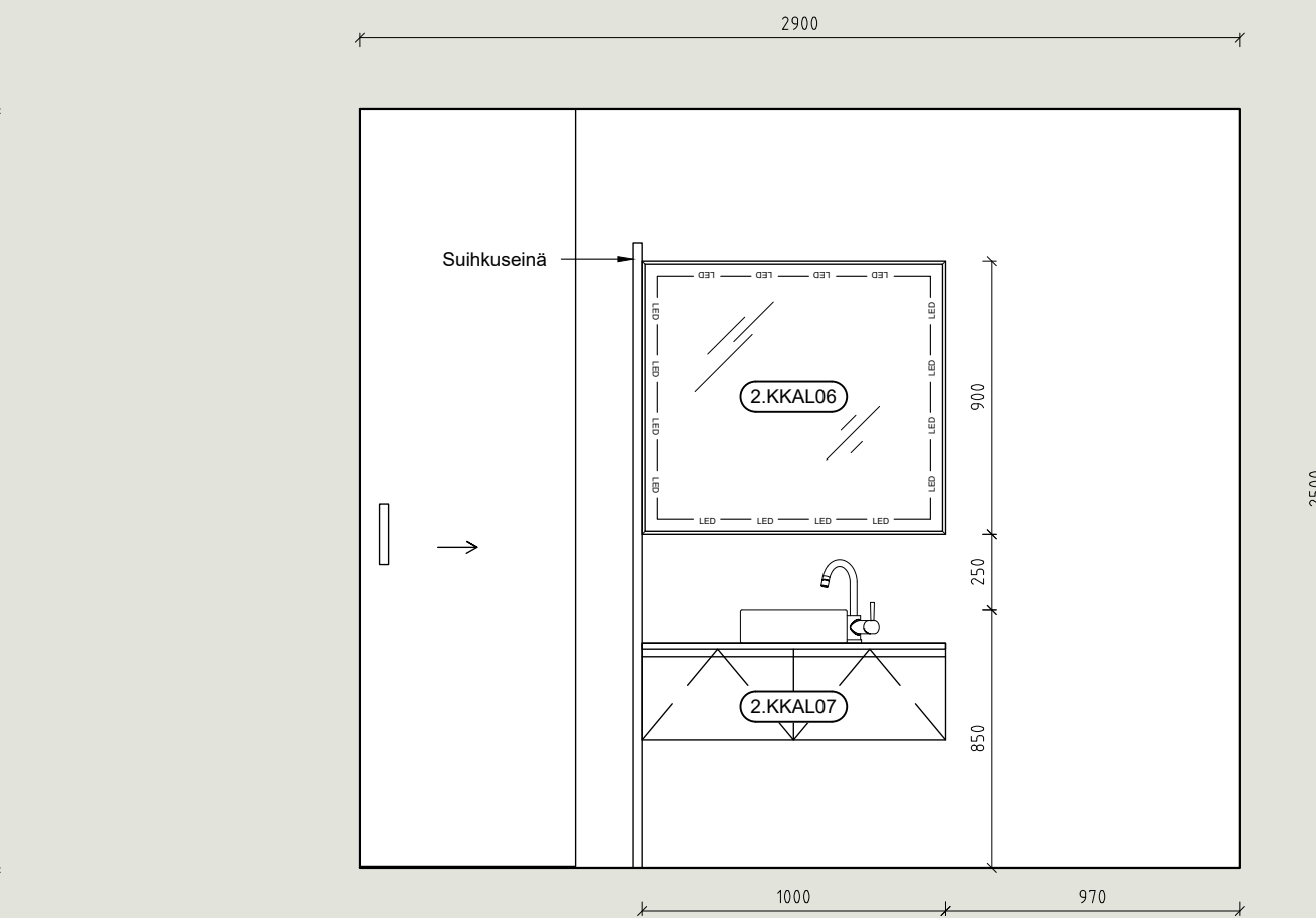
P5 M-MODUULI 1:25 Keittiö + WC
