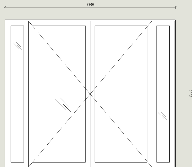
P5 S-MODUULI 1:25 Keittiö ja WC
