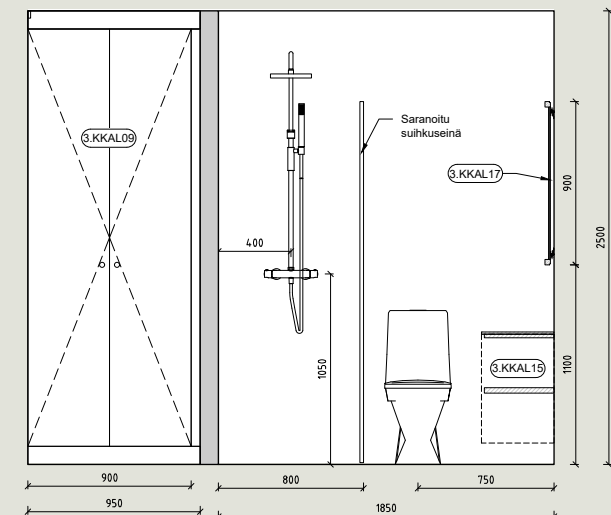
P7 Pesuhuone Helmi
