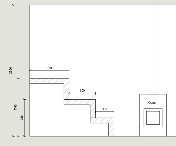
P12 Sauna Sauna 1:25
