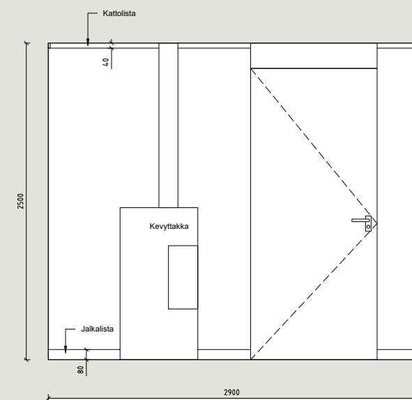
P4 Oleskelutila Sauna 1:25
