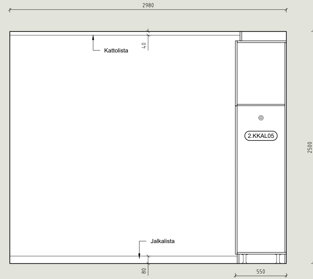
P11 M-MODUULI 1:25 Makuuhuone + WC
