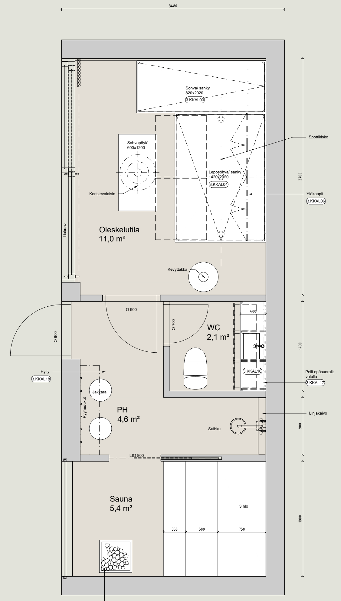
L- MODUULI SAUNA KERROSALA 30,2 m 2
