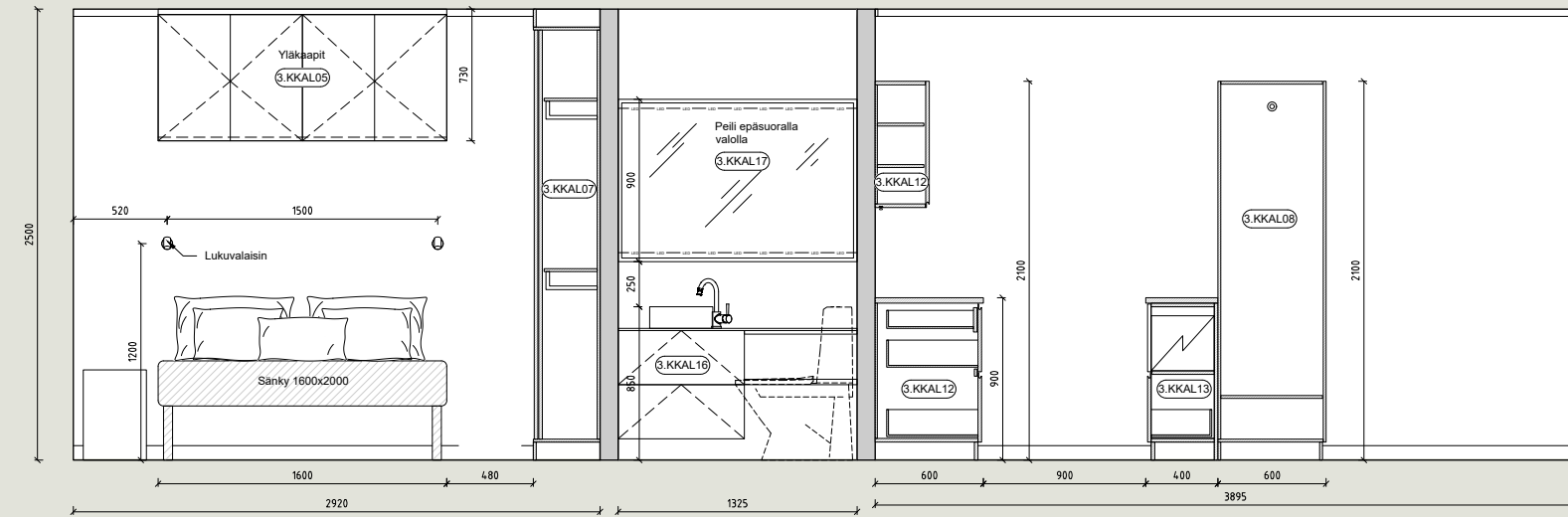
P2 Makuuhuone, WC, keittiö, oleskelutila 1:25 Army
