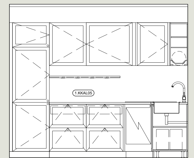
P17 S-MODUULI 1:25 Keittiö
