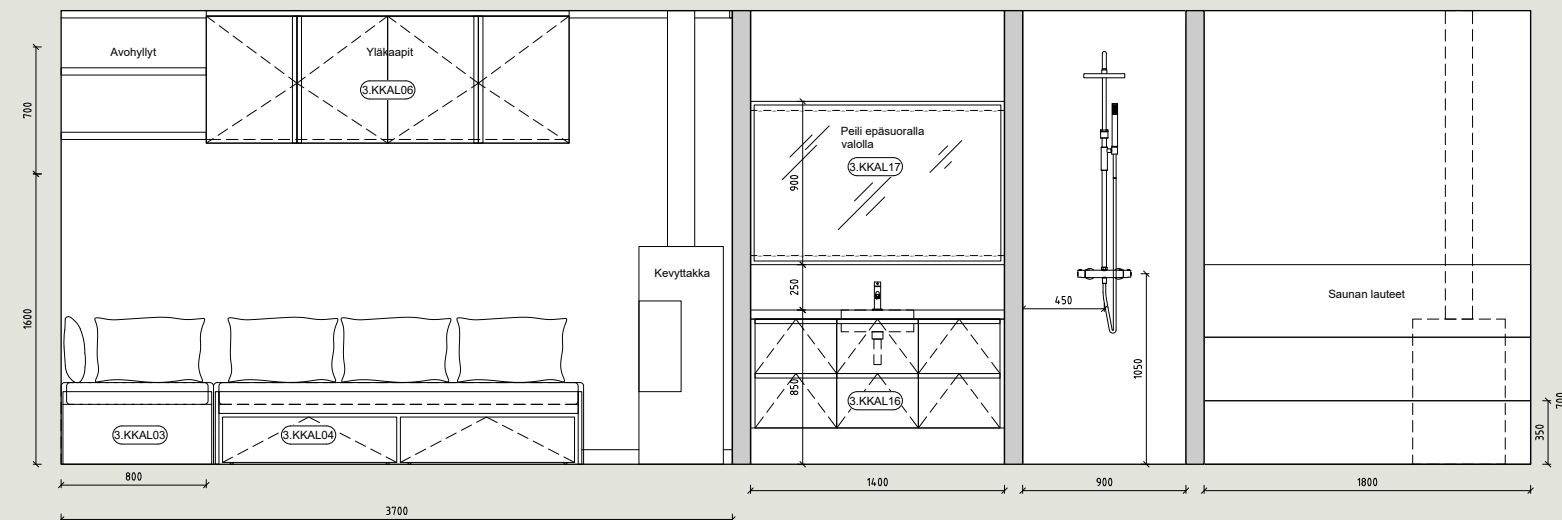
P2 Oleskelutila, WC, Sauna Sauna 1:25
