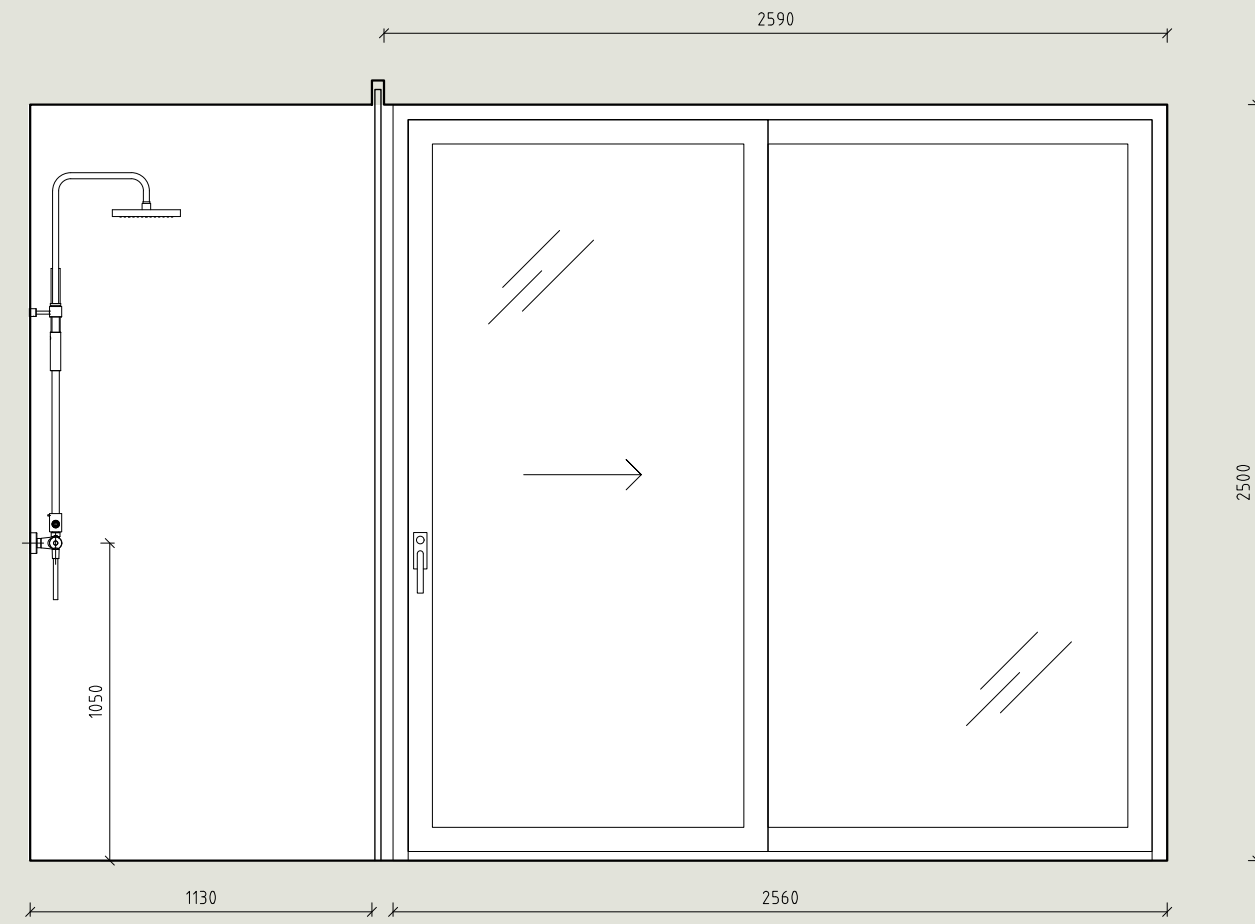
P14 M-MODUULI 1:25 Makuuhuone + WC
