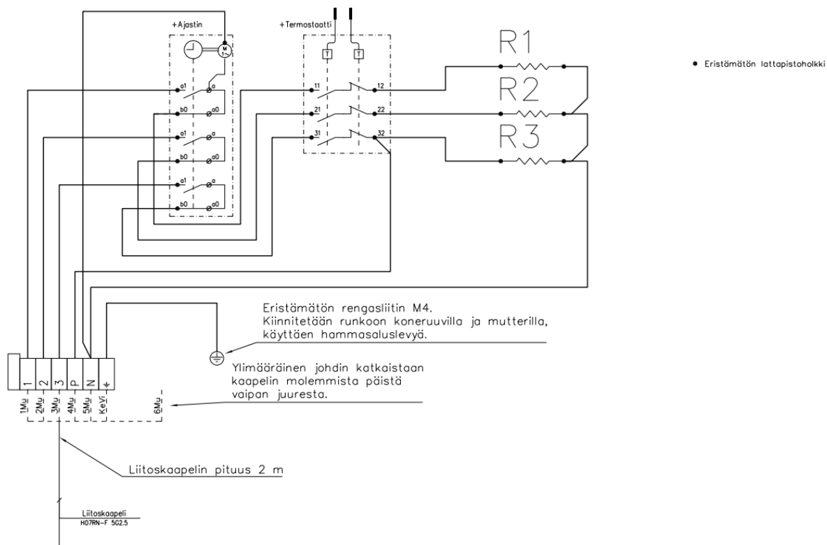
Kuva: kytkentäkaavio kiinteäohjaus
