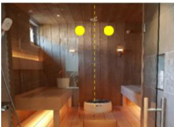
Sensorien asettelu kiukaan keskilinjan molemmiin puoliin samalle seinälle.
